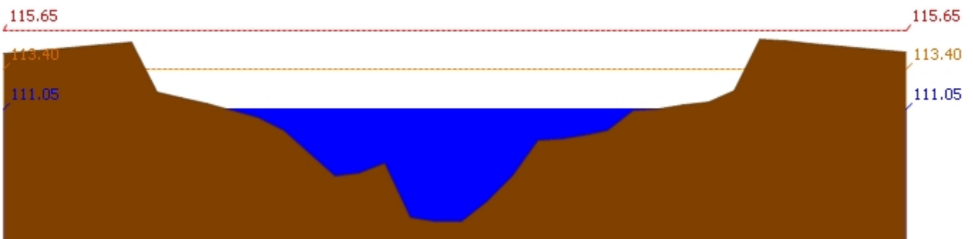
สถานี 120107T แม่น้ำป่าสักที่ อ.เมืองเพชรบูรณ์ ต.นาป่า อ.เมือง จ.เพชรบูรณ์ ระดับน้ำ 111.05 ม.รทก.
