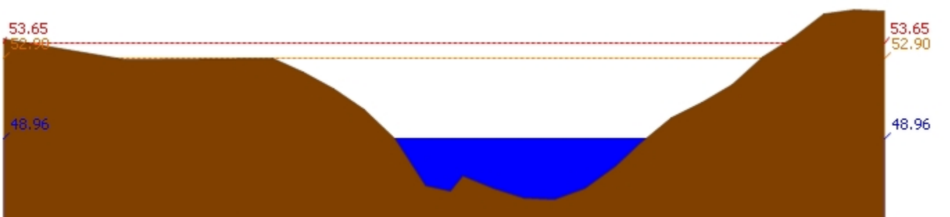
สถานี 120113T แม่น้ำป่าสักที่บ้านเขาค้าง ต.คลองกระจ้ง อ.ศรีเทพ จ.เพชรบูรณ์ ระดับน้ำ 48.96 ม.รทก.
