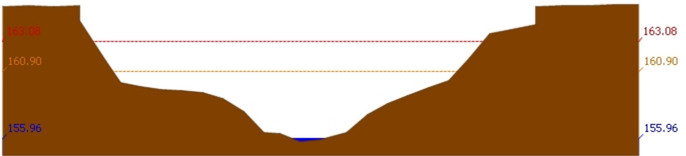
สถานี 120105T แม่น้ำป่าสักที่บ้านวังมเสหนือ ต.ทำอิบุญ อ.หล่มสัก จ.เพชรบูรณ์ ระดับน้ำ 155.96 ม.รทก.
