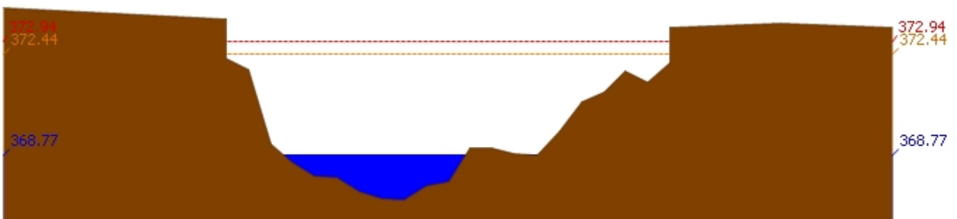
สถานี 060109T แม่น้ำปิงที่บ้านสบอ้อ ต.แม่่นะ อ.เชียงดาว จ.เชียงใหม่ ระดับน้ำ 368.77 ม.รทก.
