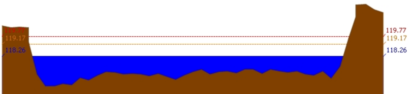
สถานี 060111T แม่น้ำปิงที่บ้านปากร่องห้วยจี้ ต.ตากออก อ.บ้านตาก จ.ตาก ระดับน้ำ 118.26 ม.รทก.
