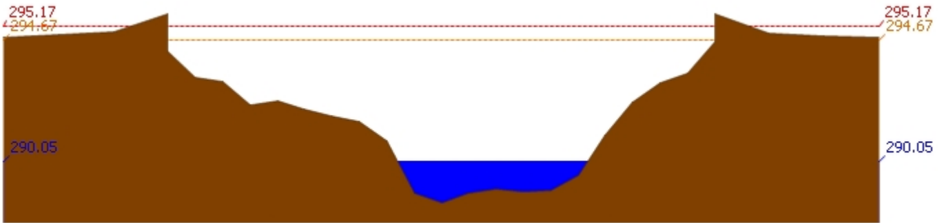
สถานี 060709T น้ำแม่กวงที่ลำพูน ต.เวียงของ อ.เมือง จ.ลำพูน ระดับน้ำ 290.05 ม.รทก.
