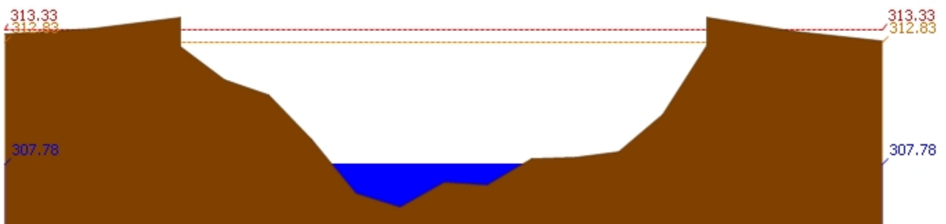
สถานี 060814T น้ำแม่ขานที่บ้านท่าโป่ง ต.บ้านแม อ.สันป่าตอง จ.เชียงใหม่ ระดับน้ำ 307.78 ม.รทก.
