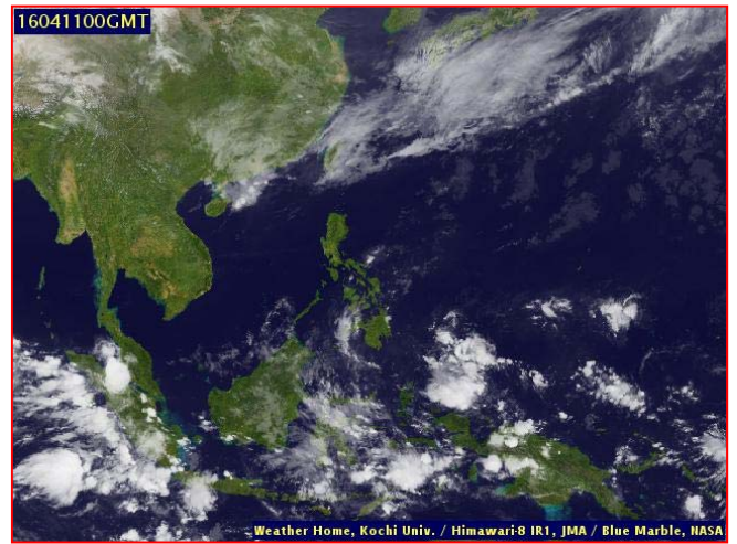
ภาพถ่ายจากดาวเทียม วันที่ ๑๑ เม.ย. ๒๕๕๙ เวลา ๐๗.๐๐ น.
