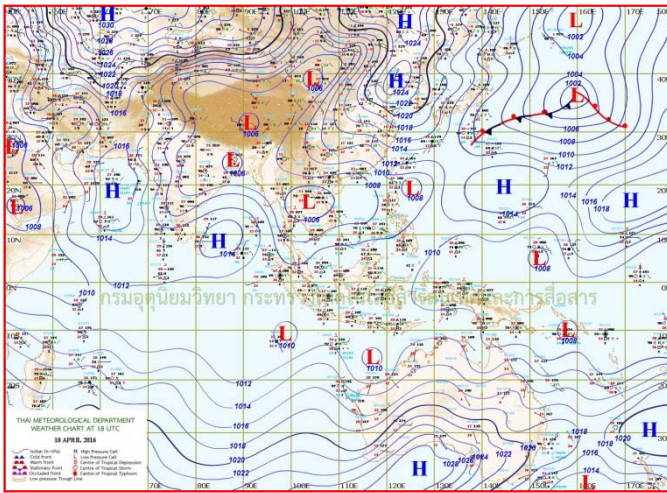
แผนที่อากาศ วันที่ ๑๑ เม.ย. ๒๕๕๙ เวลา ๐๖.๐๐ น.
