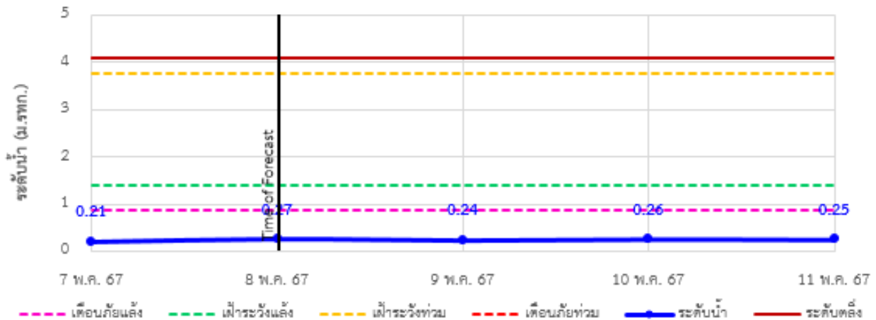
TC191913 สะพานคีรีวง ต.ท่าโลน อ.ลานสกา จ.นครศรีธรรมราช
