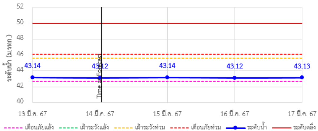
TC191913 สะพานคีรีวง ต.กำไล อ.ลานสกา จ.นครศรีธรรมราช
