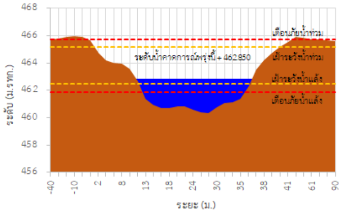
TC030114 สะพานพ่อยุเมืองรามมหาราช
