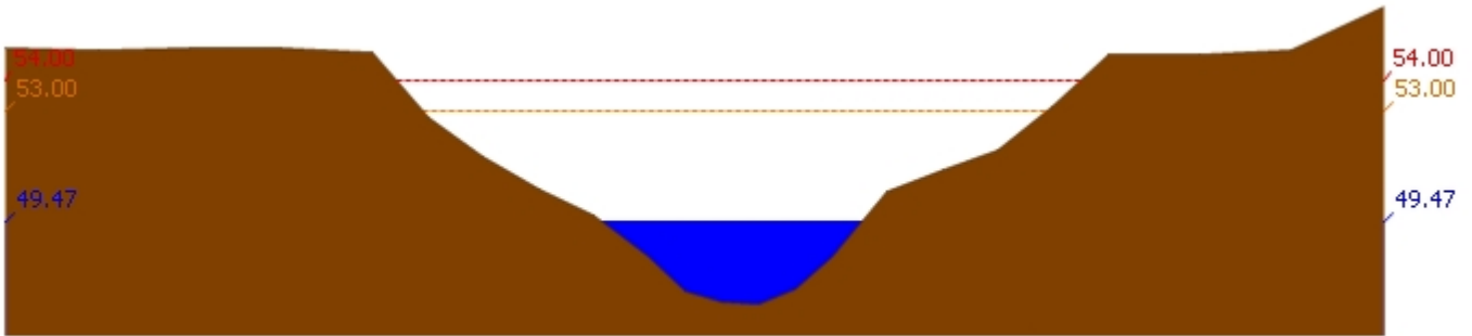
สถานี 120702T ลำสนธิที่บ้านท่าช้าง ต.หนองขาหย่าง อ.ชัยบาดาล จ.ลพบุรี ระดับน้ำ 49.47 ม.รทก.
