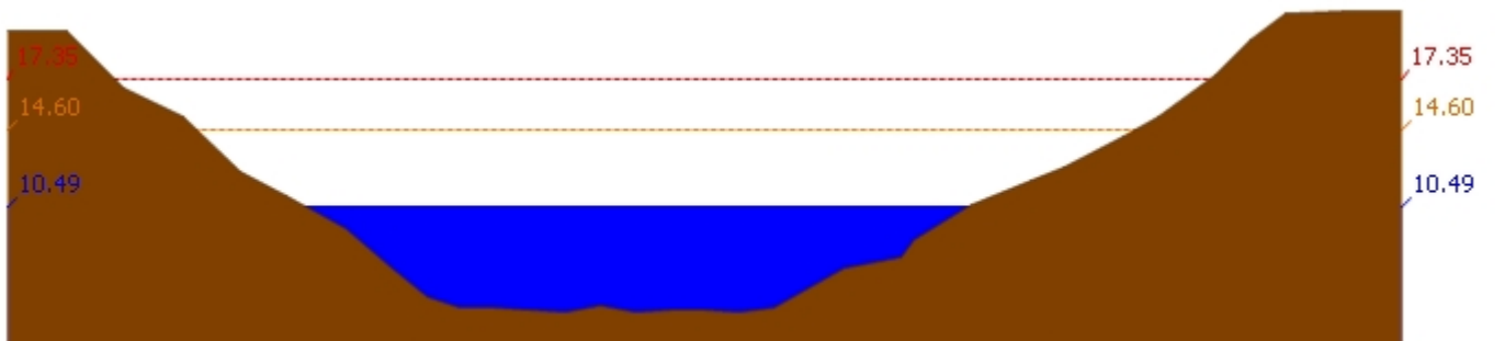
สถานี 120109T แม่น้ำป่าสักที่ อ.แก่งคอย ต.แก่งคอย อ.แก่งคอย จ.สระบุรี ระดับน้ำ 10.49 ม.รทก.
