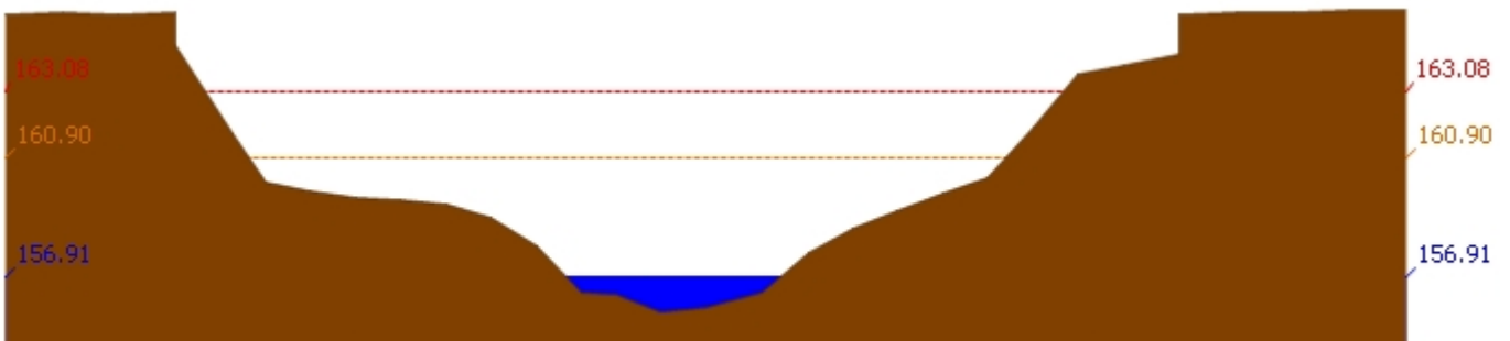
สถานี 120105T แม่น้ำป่าสักที่บ้านวังมเหนื่อ ต.ท่าอิฐ อ.หล่มสัก จ.เพชรบูรณ์ ระดับน้ำ 156.91 ม.รทก.
