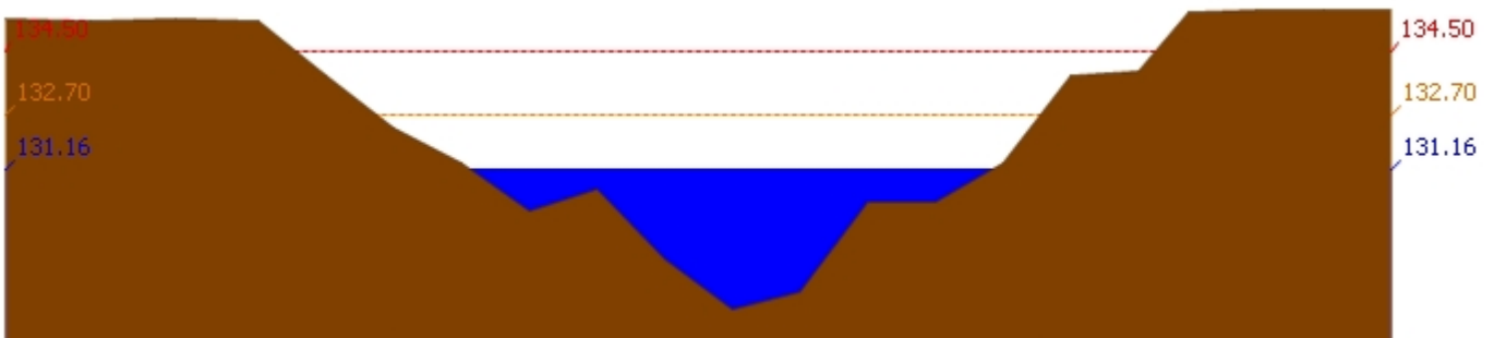
สถานี 120111T แม่น้ำป่าสักที่บ้านจางวาง ต.ลานบัว อ.หล่มสัก จ.เพชรบูรณ์ ระดับน้ำ 131.16 ม.รทก.
