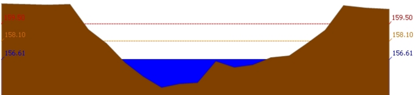
สถานี 120305T หัวน้ำพุที่ อ.หล่มเก่า ต.หล่มเก่า อ.หล่มเก่า จ.เพชรบูรณ์ ระดับน้ำ 156.61 ม.รทก.
