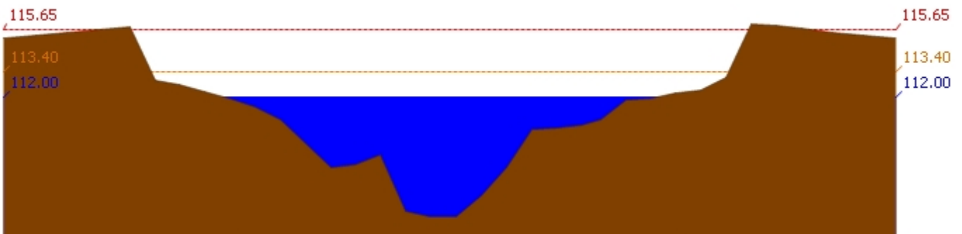
สถานี 120107T แม่น้ำป่าสักที่ อ.เมืองเพชรบูรณ์ ต.นาป่า อ.เมือง จ.เพชรบูรณ์ ระดับน้ำ 112.00 ม.รทก.
