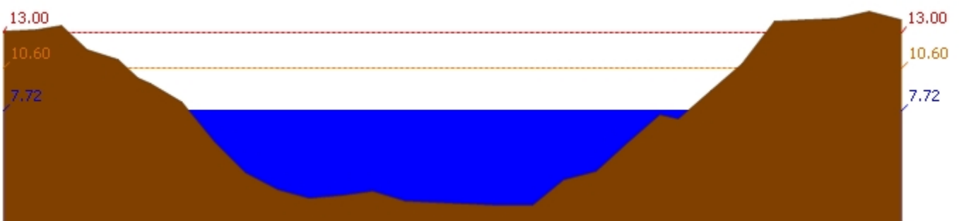
สถานี 120106T แม่น้ำป่าสักที่ อ.เสนาห์ ต.ศาลาวิไทย อ.เสนาห์ จ.สระบุรี ระดับน้ำ 7.72 ม.รทก.
