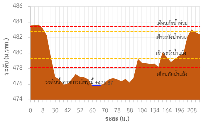
TC010509 สะพานข้ามคลองแม่เลี้ยง
