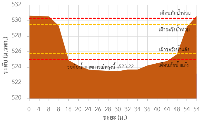
TC011008 สะพานบ้านคองฝั้ง - บ้านห้วยสิงห์
