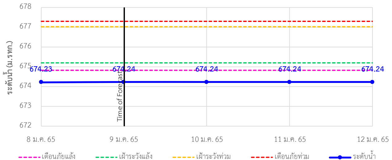
TC010605 สะพานบ้านป่าปู้ ต.ผาป่อง อ.เมือง จ.แม่ฮ่องสอน
