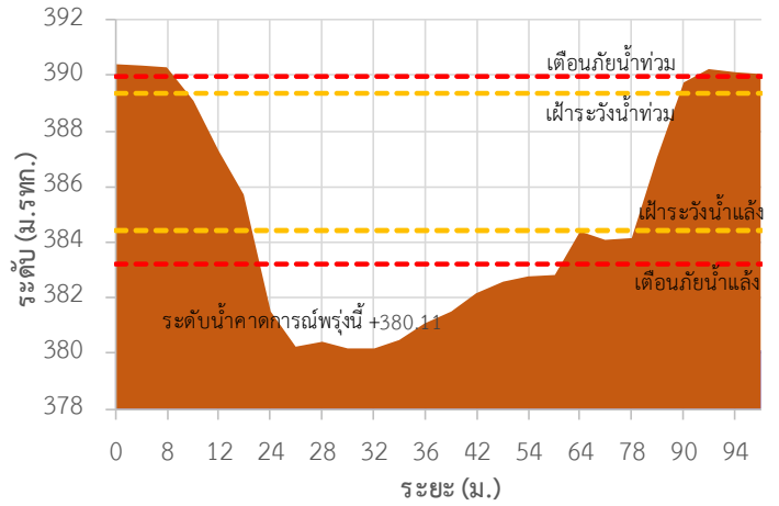
TC011009 สะพานร่วมใจบ้านท่าผาป๋ม
