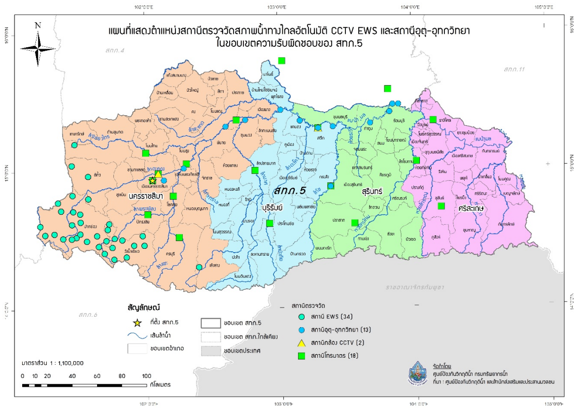
รูปที่ 4 ตำแหน่งสถานีตรวจวัดสภาพน้ำทางไกลอัตโนมัติ CCTV EWS และสถานีอุตุ-อุทกวิทยา ในเขตพื้นที่ความรับผิดชอบของสำนักงานทรัพยากรน้ำภาค 5
